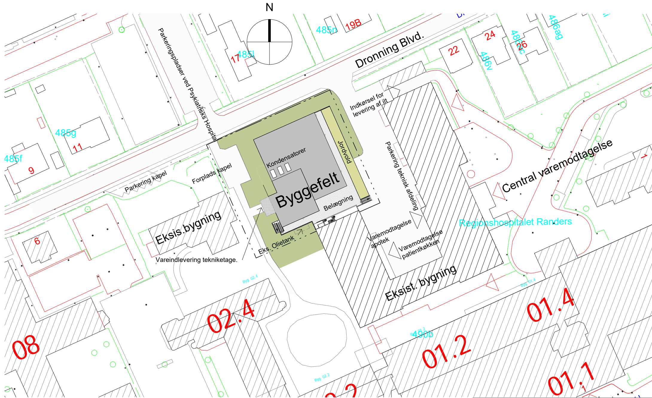
Situationsplan | 1 : 1000
