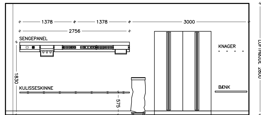
OPSTALT B-B
