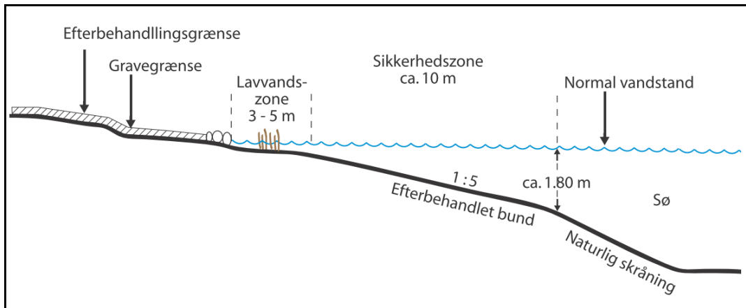
Figur 1a: Principskitse for efterbehandling af gravesø.
