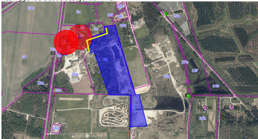
Figur 1 Principiel placering af 3 m høje jord/støjvolde. Voldene er vist med lilla, tilladelsesarealet med gennemsigtigt grøn flade. Røde cirkler viser tilladelsens afstandskrav til drikkevandsboringer (min. 75 meter).
