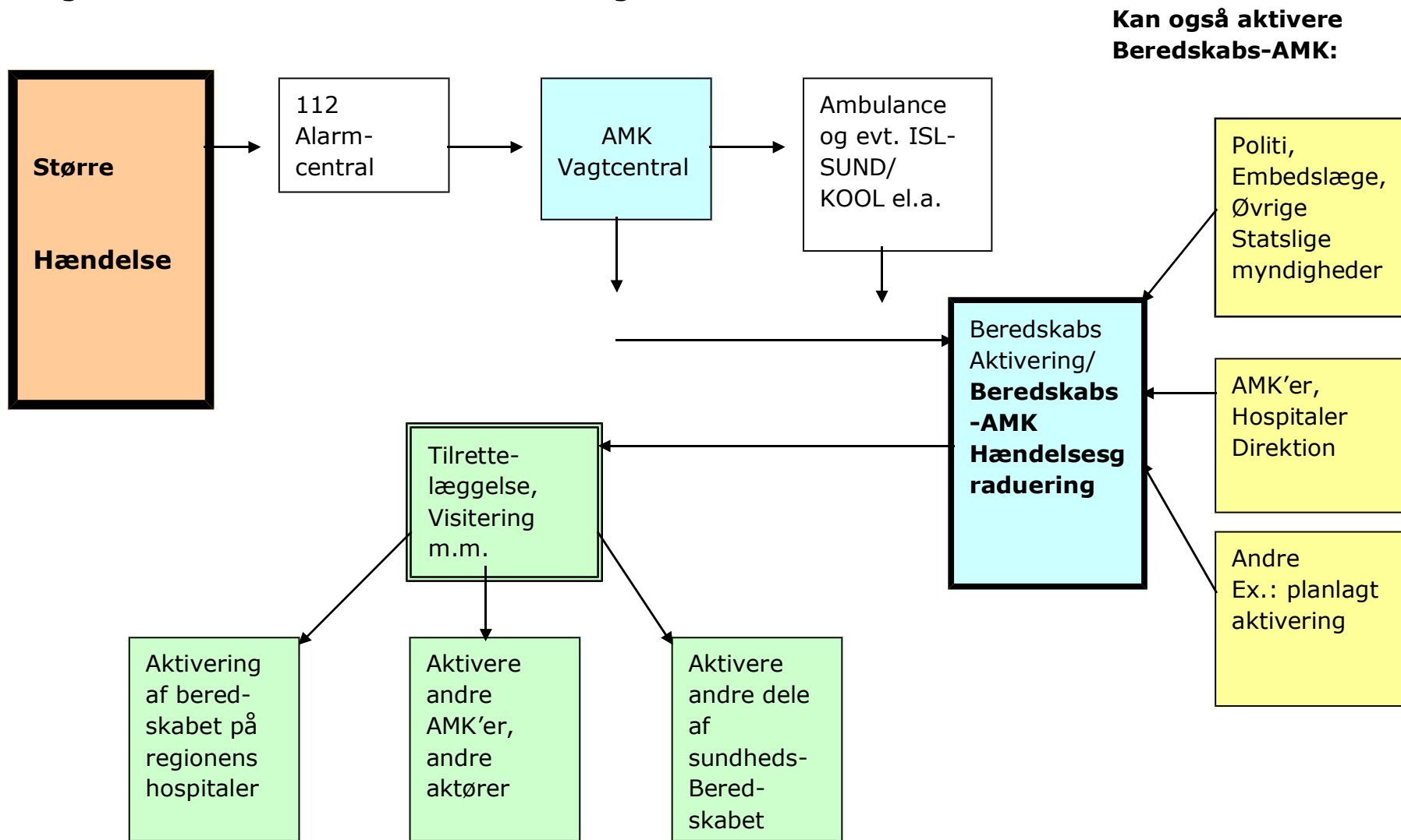
Figur 3: Sundhedsberedskabets aktivering
