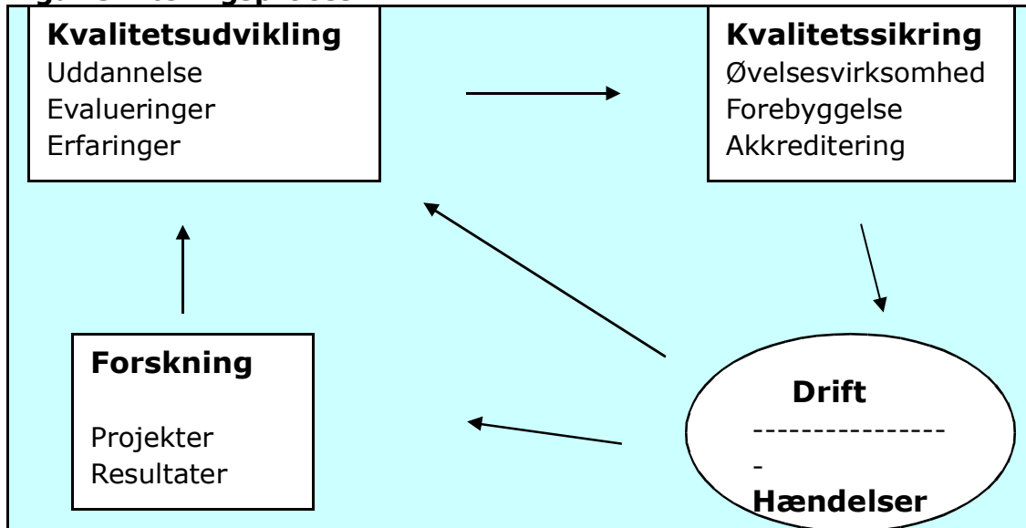
Figur 5: Læringsproces
