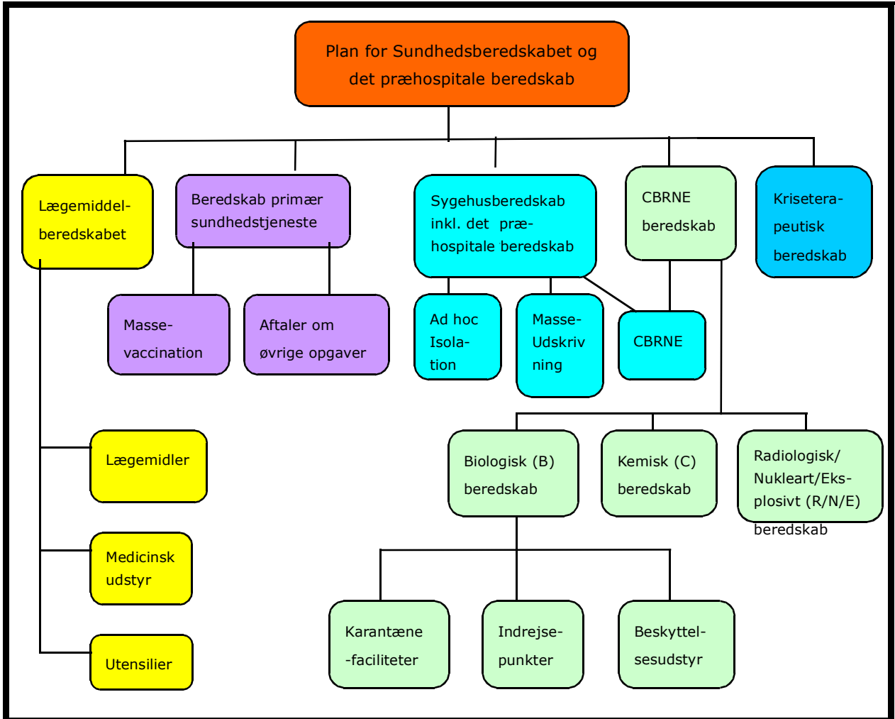
Figur 1: Planelementer
