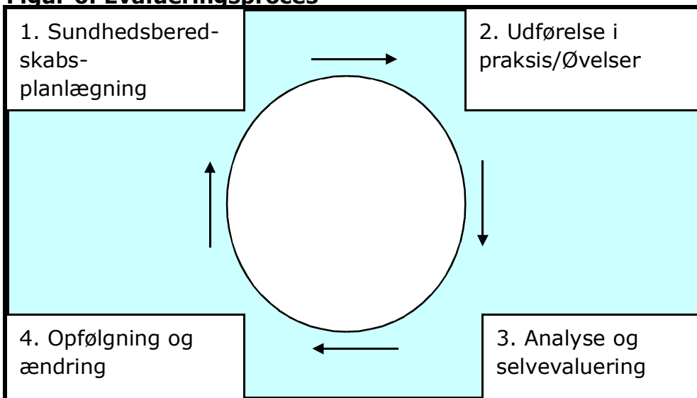
Figur 6: Evalueringsproces
